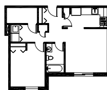
Type D-1cc 57 m 2
