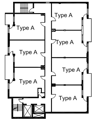
Étage type
