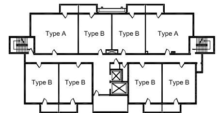
Étage type
